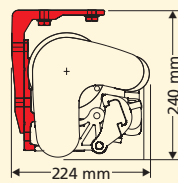
Deckenmontage
