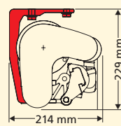
Deckenmontage, kompakt
