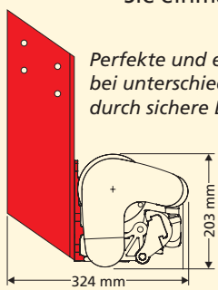
Dachsparrenmontage
